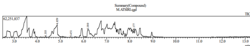
Gambar 1. Kromatografi Gas
