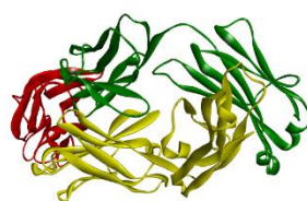
Gambar 3. Struktur Kristal 4G3Y
